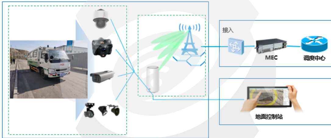
图 4.7 测试床 5G 井下无轨胶轮车无人驾驶应用方案
